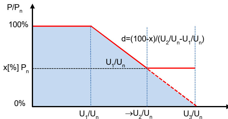
Obr. 19 Charakteristika funkce P(\underline{U})
