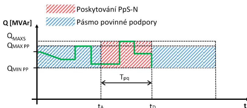
Obr. 10 Příklad hodnocení služby jalového výkonu řízení toků jalových výkonů pro nově připojované výrobní moduly
