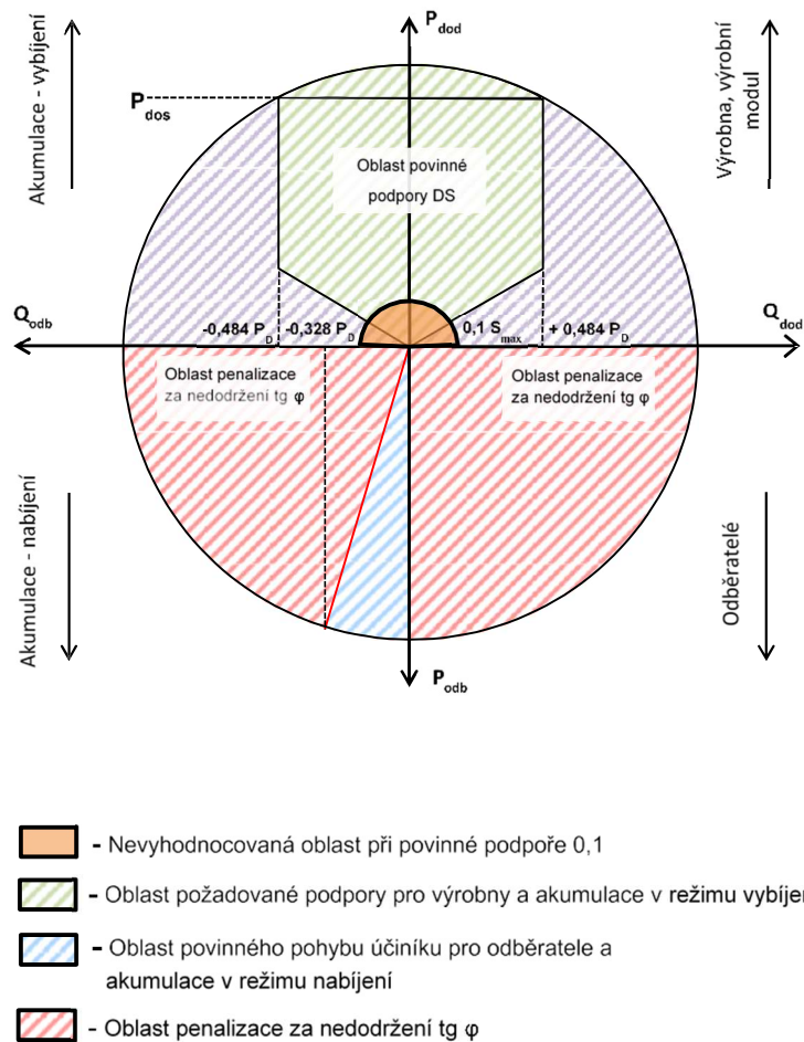
Obr. 1 Požadavky povinné podpory výroben/výrobních modulů a odběratelů
