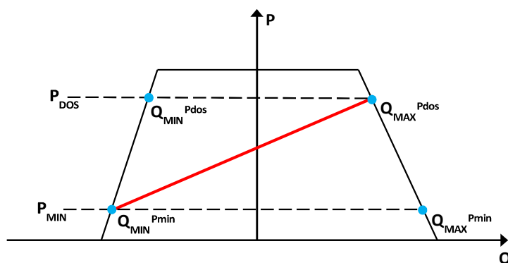
Obr. 6 Certifikovaný rozsah jalového výkonu
