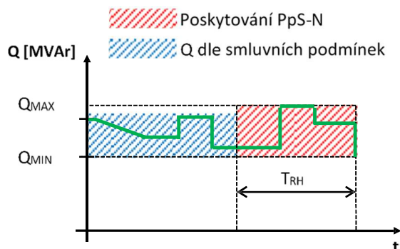
Obr. 9 Příklad hodnocení služby jalového výkonu řízení napětí pro stávající výrobní
