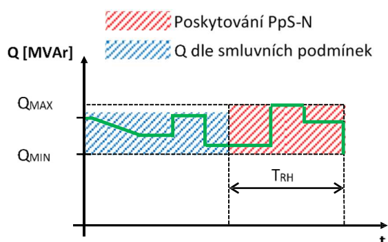
Obr. 12 Příklad hodnocení služby jalového výkonu řízení toků jalových výkonů pro stávající výrobní
